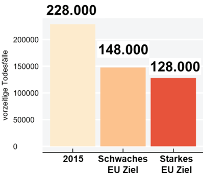
Abbildung 5: Anzahl der durch Luftverschmutzung verursachten vorzeitigen Todesfälle in Abhängigkeit des EU-Klimaschutzziels (Potsdam-Institut für Klimafolgenforschung)
