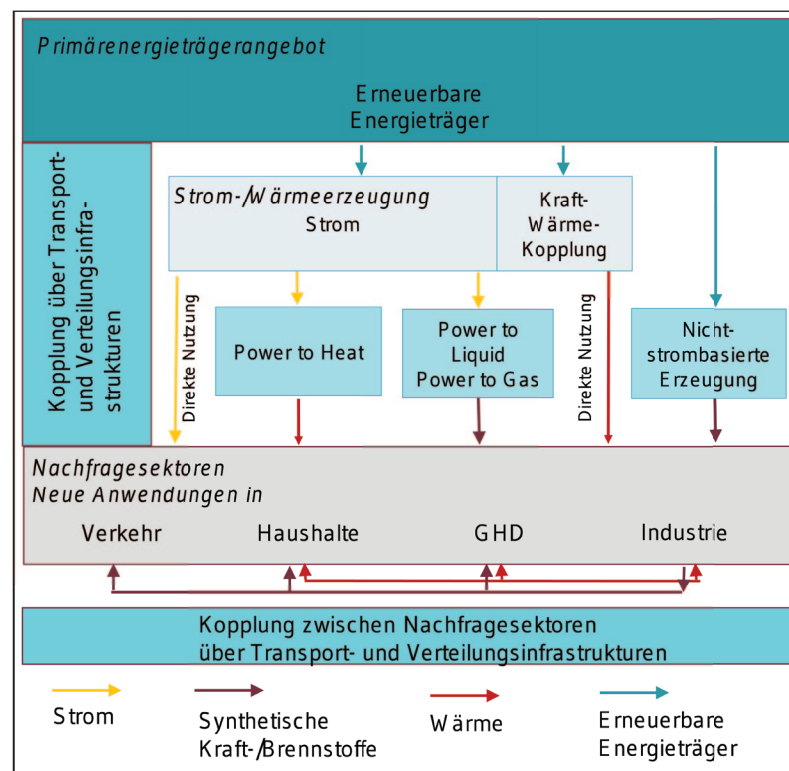
Abbildung 7: Verbindung der Sektoren ist eine der zentralen Aufgaben der Energiewende (Fraunhofer-Institut für Solare Energiesysteme ISE)
