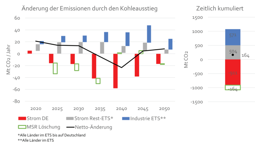
Abbildung 4: Differenz der Emissionen zwischen den Szenarien „Kohleausstieg“ und „Referenz (kein Ausstieg)“ (Potsdam-Institut für Klimafolgenforschung)
